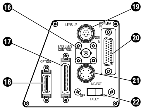
Drehkopf-Anschlussstafel
