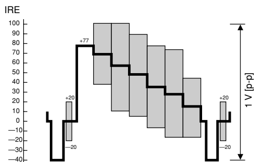
Oszilloskop (FBAS-Signale)
